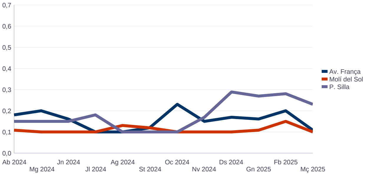
Contaminación atmosférica media mensual por monóxido de carbono Contaminació atmosfèrica mitjana mensual per monòxid de carboni
