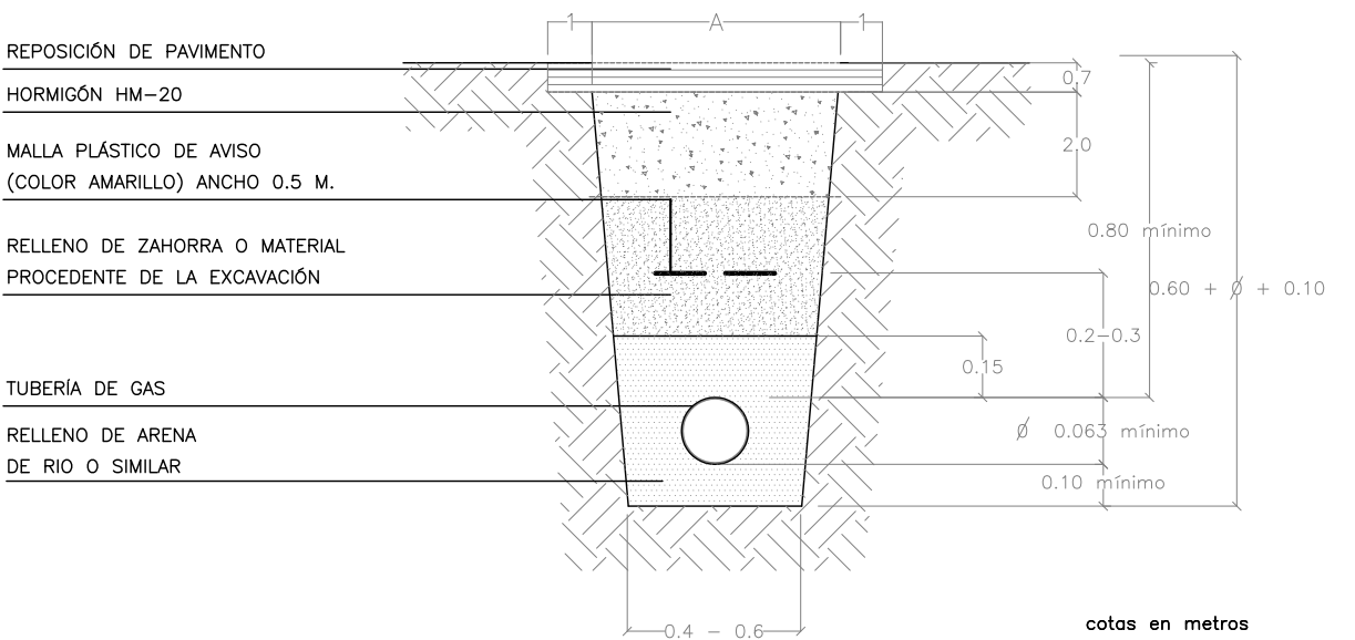
ZANJA TIPO PARA CANALIZACIÓN DE GAS EN CALZADA
