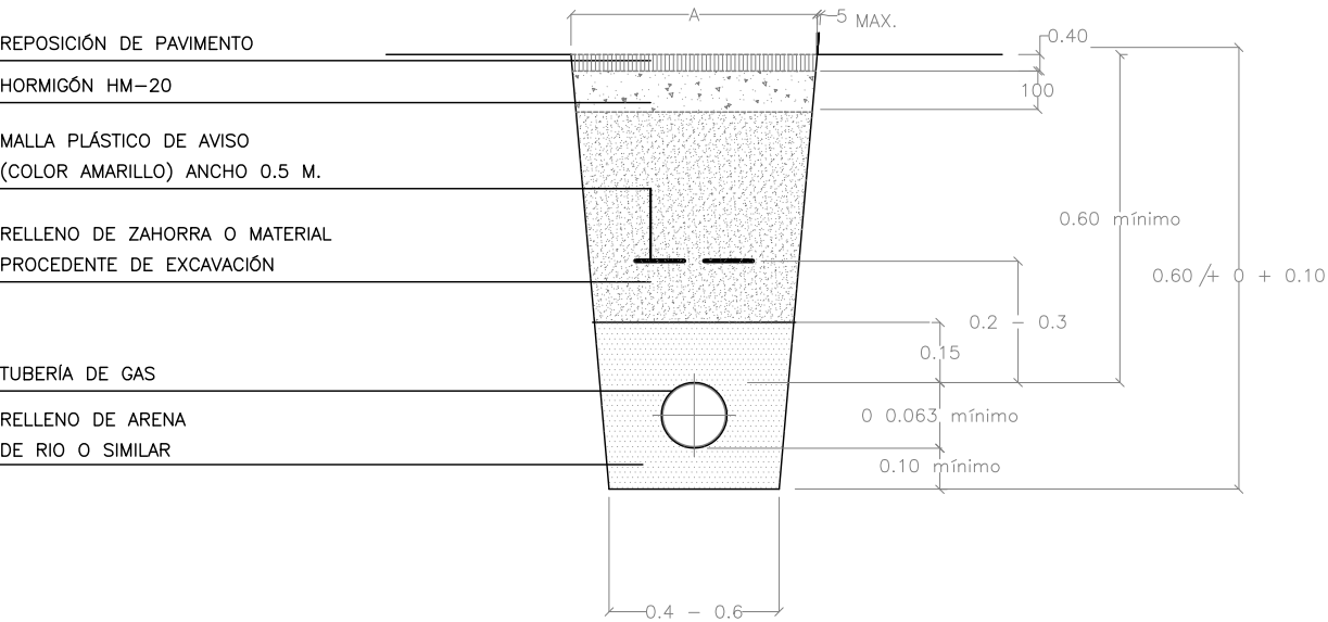
ZANJA TIPO PARA CANALIZACIÓN DE GAS EN ACERA
