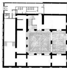
PLANTA BAJA
