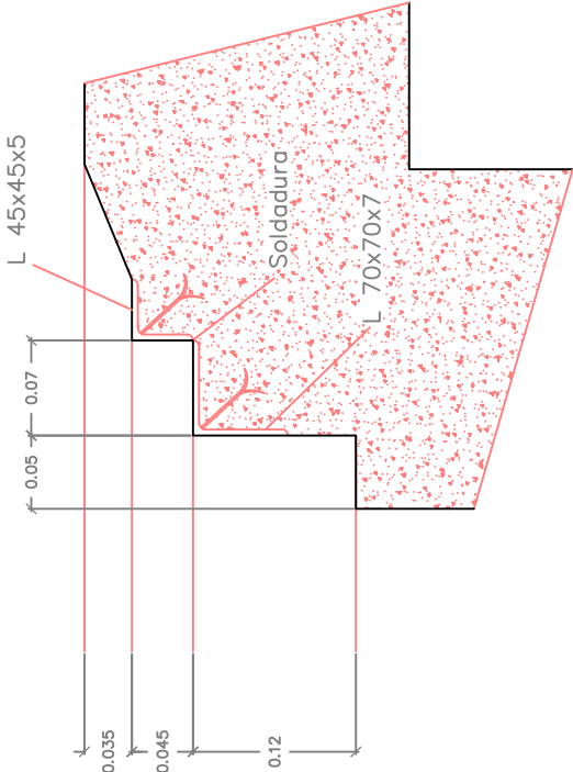
detalle C
