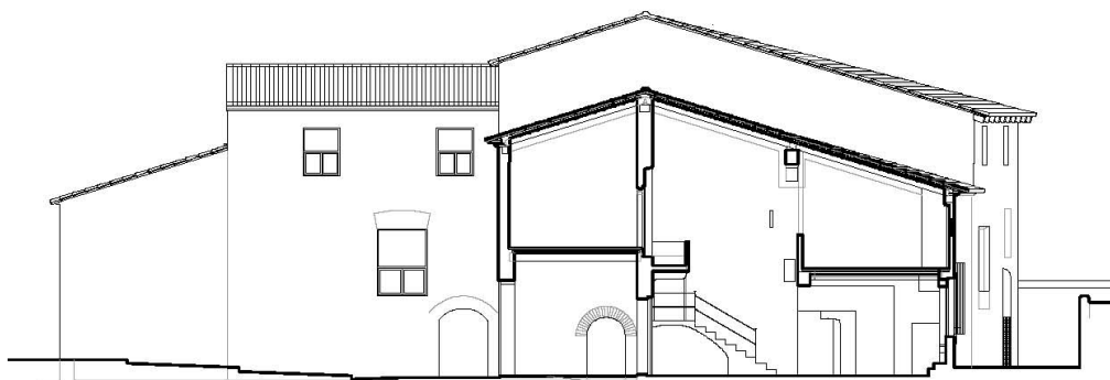
SECCION LONGITUDINAL
