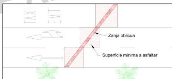
Figura 2. Afecció diversos carrils. Superfície mínima.
