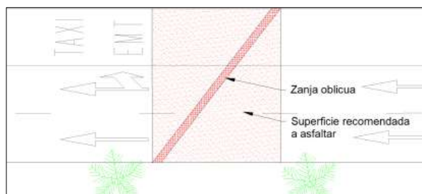
Figura 3. Afecció diversos carrils. Superfície recomanada.
