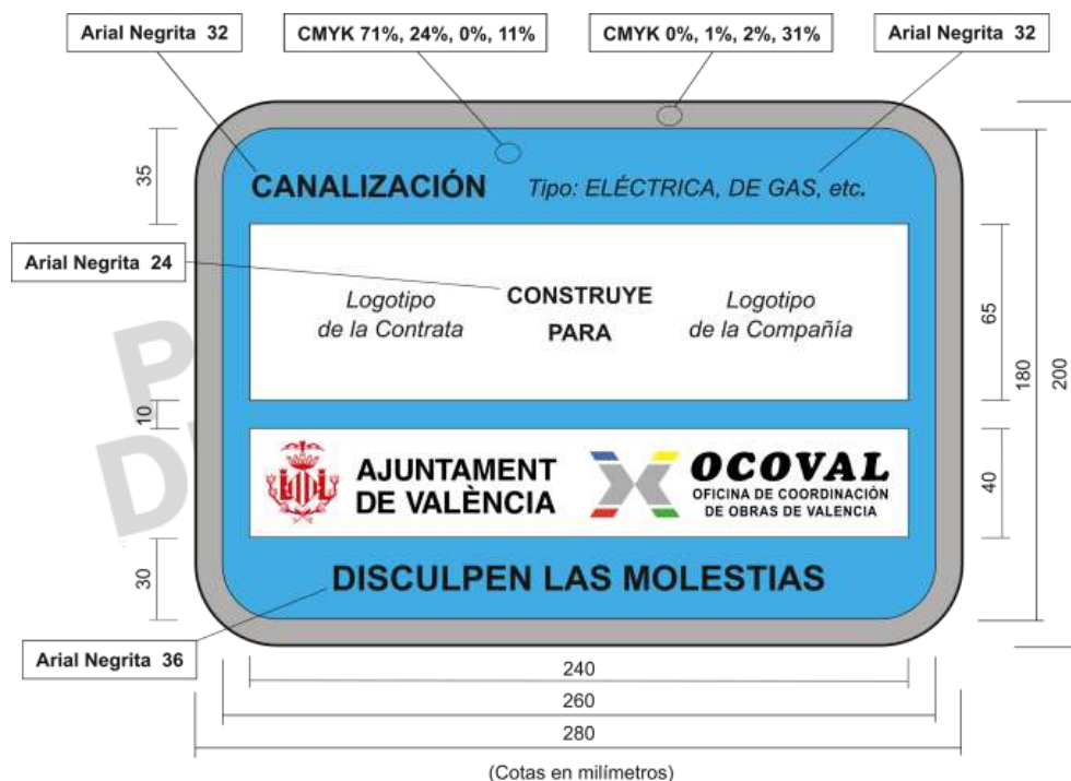
Figura 2. Cartell d'obra per a col·locació en tanques
