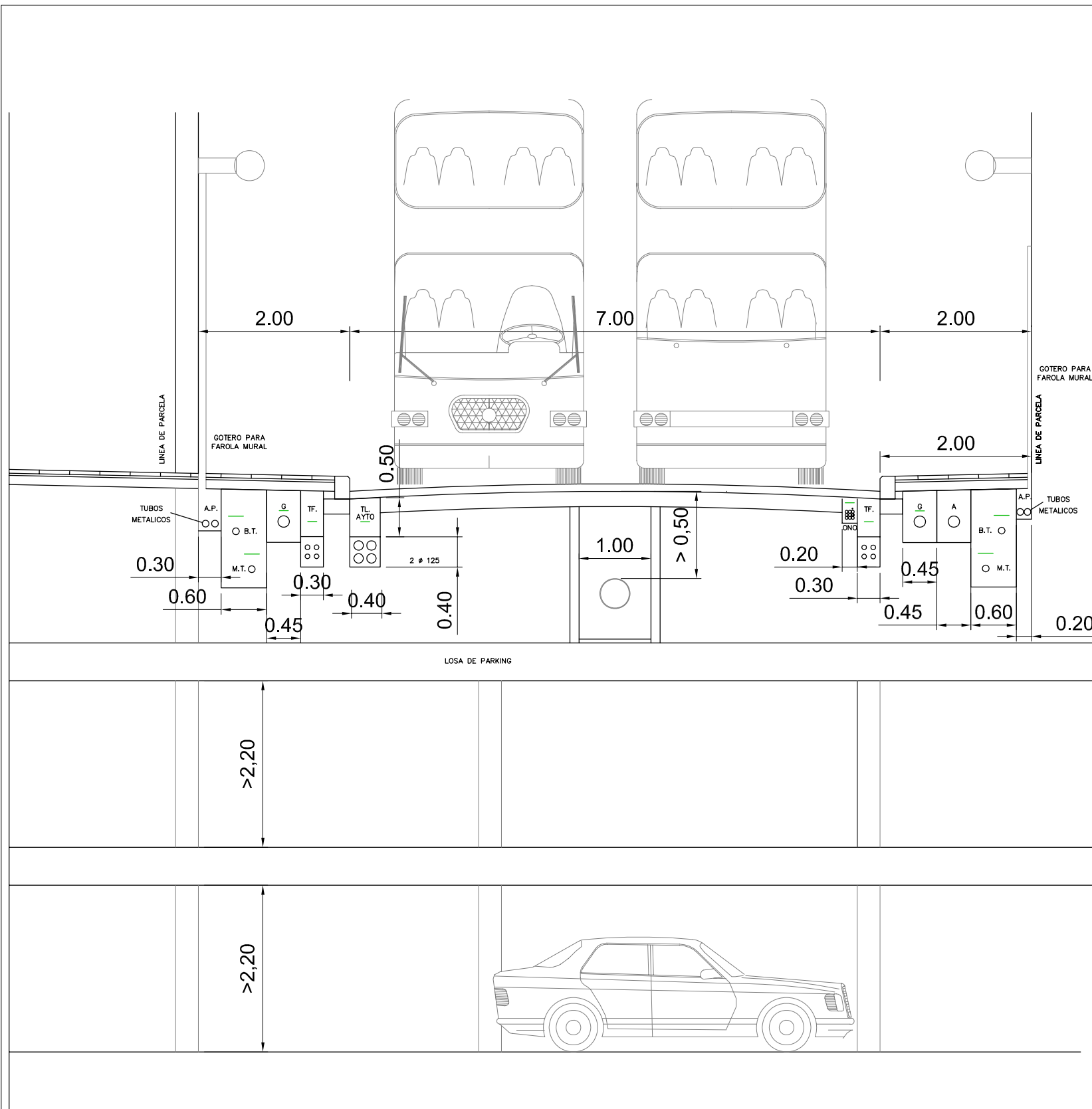
SECCIÓN TIPO CALLE BOTELLAS
