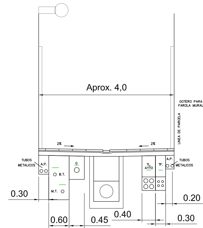
SECCIÓN TIPO CALLES PEATONALES
