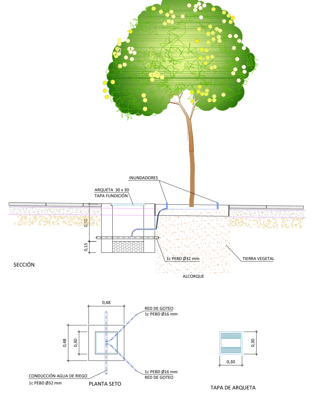
DETALLE ARQUETA ESCALA 1/30
