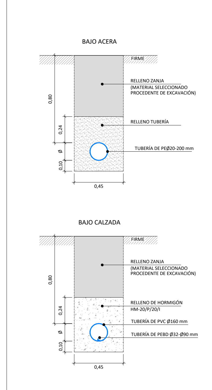
ZANJA DE RIEGO ESCALA 1/10
