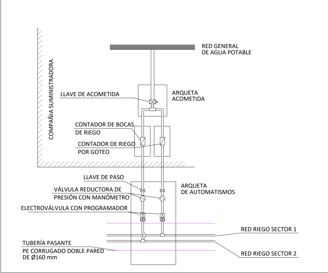
ESQUEMA RED S/E
