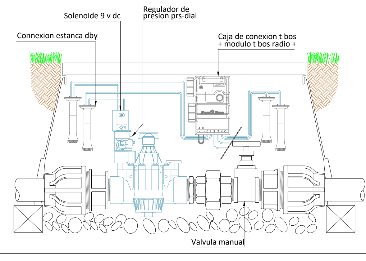
ELECTROVÁLVULA PGA / T BOS S/E
