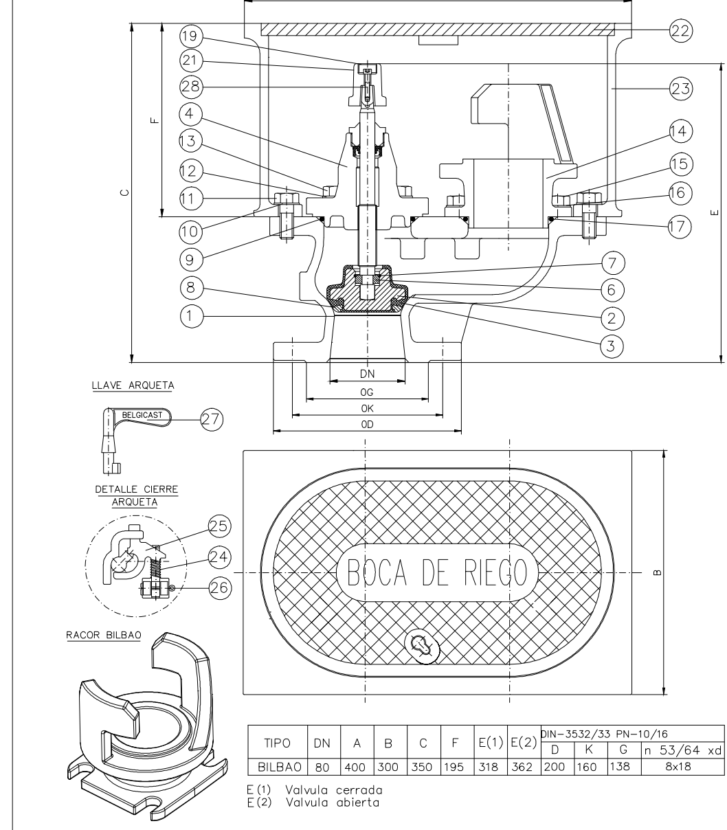
BOCA DE RIEGO ESCALA 1/10
