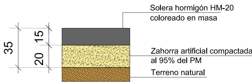
P13 - CARRIL BICI SOLERA HORMIGÓN
