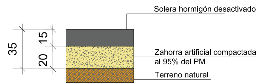
P10 - CAMINO PEATONAL HORMIGÓN DESACTIVADO
