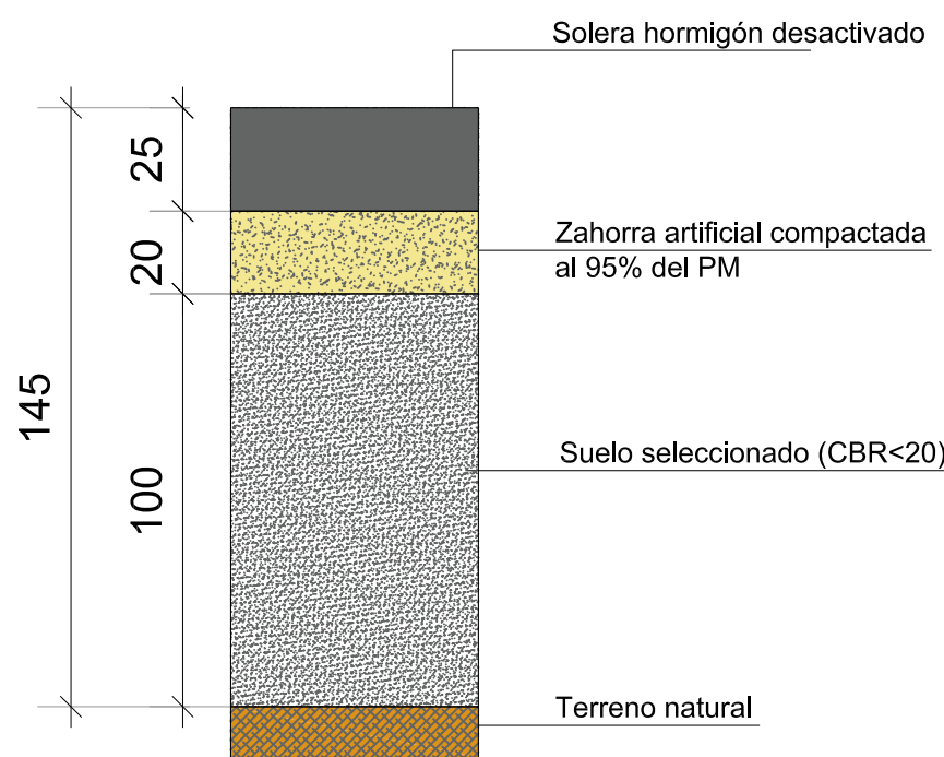
P11 - CAMINO RODADO HORMIGÓN DESACTIVADO (BOMBEROS)
