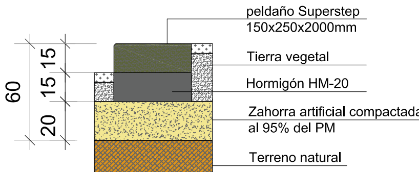
P17 - GRADERÍO PELDAÑO PREFABRICADO
