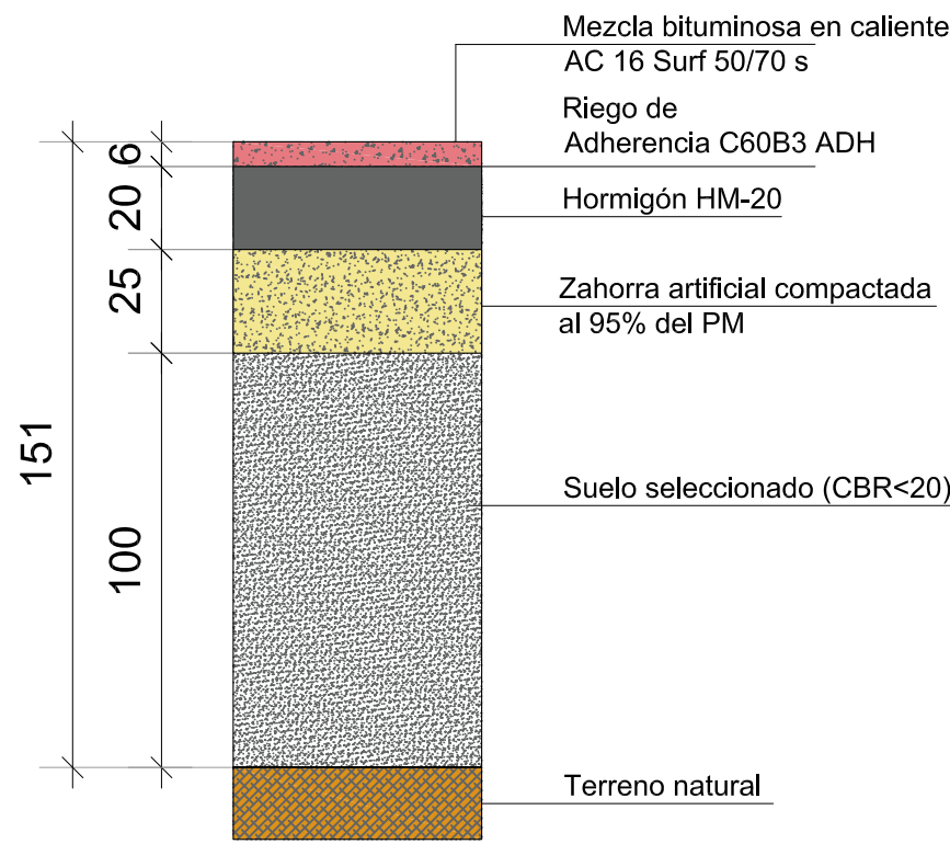
P01 - CALZADA ESTÁNDAR
