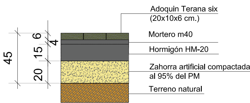
P07 - ACERA ADOQUÍN TRÁFICO PEATONAL
