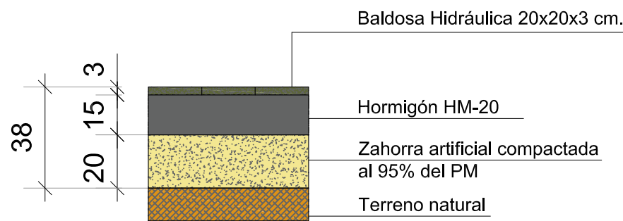
P03 - ACERA BALDOSA 20x20
