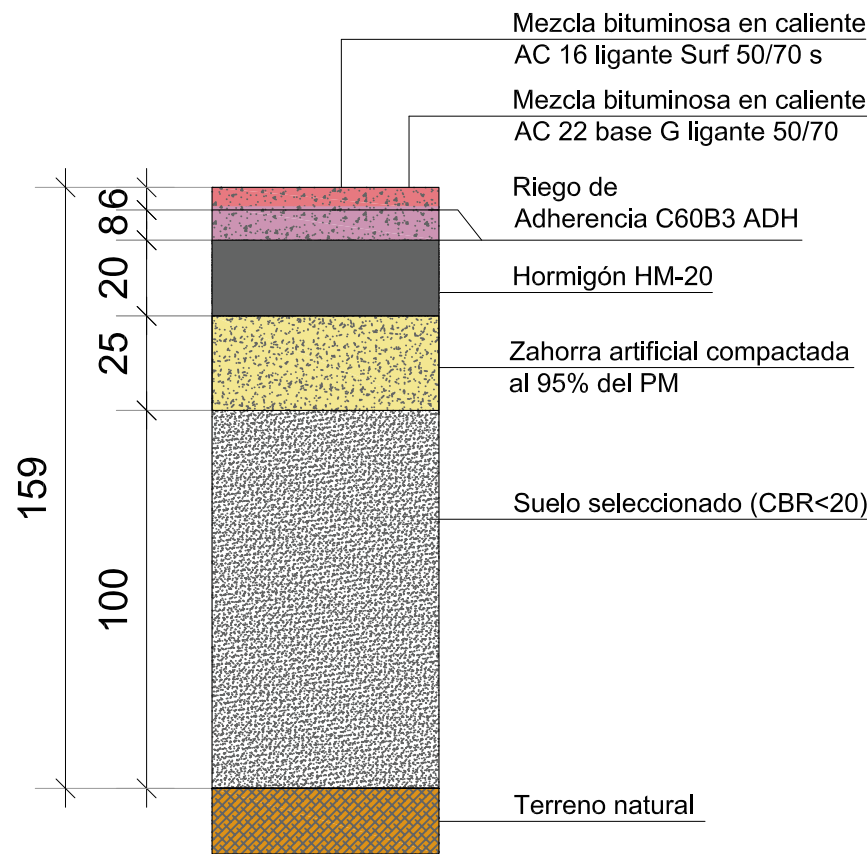
P02 - CALZADA RONDA (CARRIL BUS)
