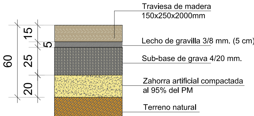
P16 - CAMINO DE TRAVIESAS DE MADERA
