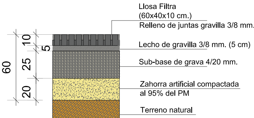
P09 - ACERA LOSA FILTRANTE PEATONAL
