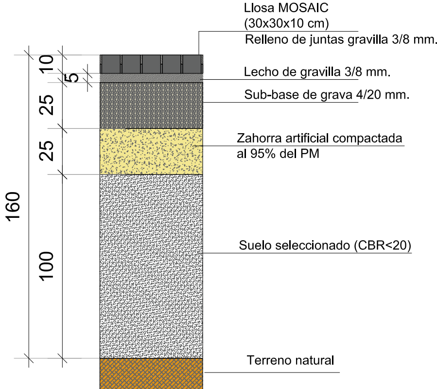
P05 - APARCAMIENTO LOSA FILTRANTE
