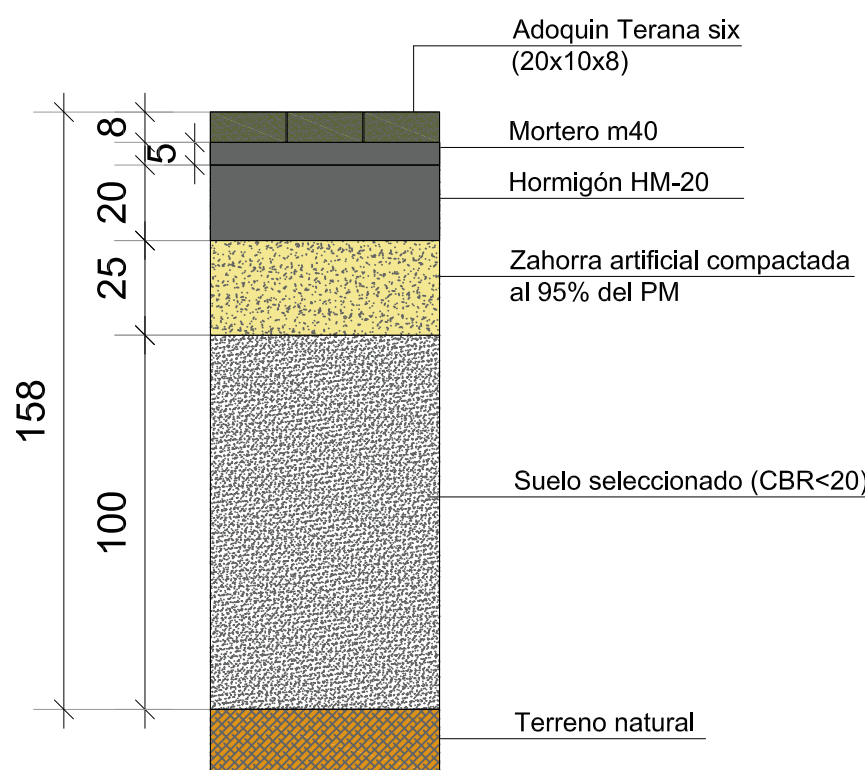
P06 - CALZADA ADOQUÍN TRÁFICO RODADO
