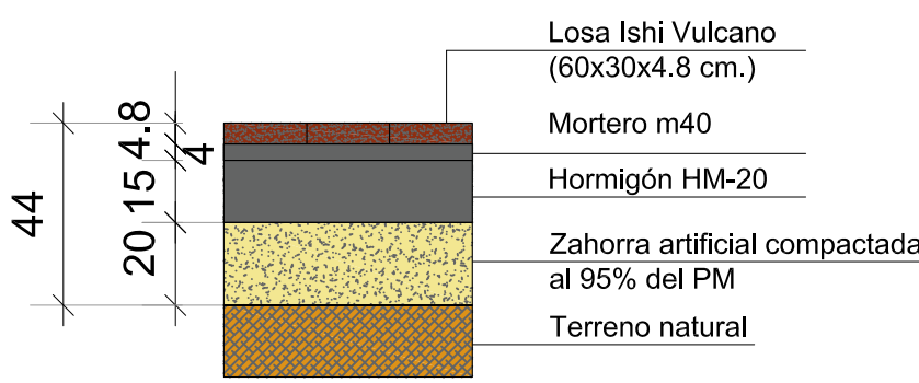
P08 - ACERA LOSA TRÁFICO PEATONAL
