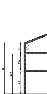
2 PLANTAS
