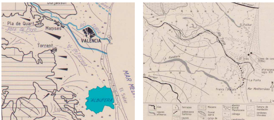
Unitats fisiogràfiques de la plana litoral Valenciana (P.Carmona) i Trets geomorfològics de la plana Valenciana. Font: Llibre Història, Geografia i Art de la Ciutat de València, tom II pàg 22. Universitat de València
