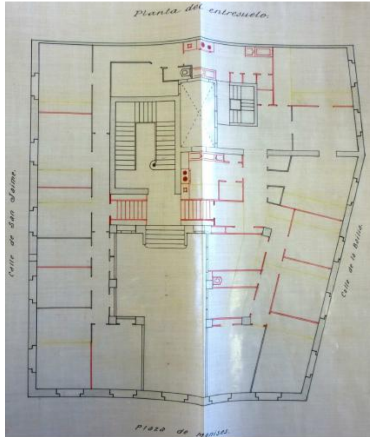
Plano del proyecto modificado. 1926
