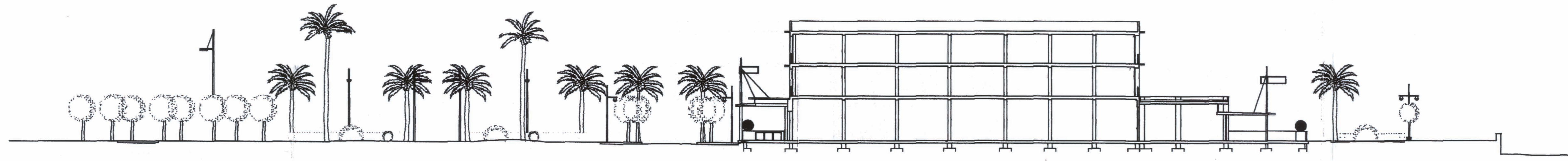
SECCION A-A'
