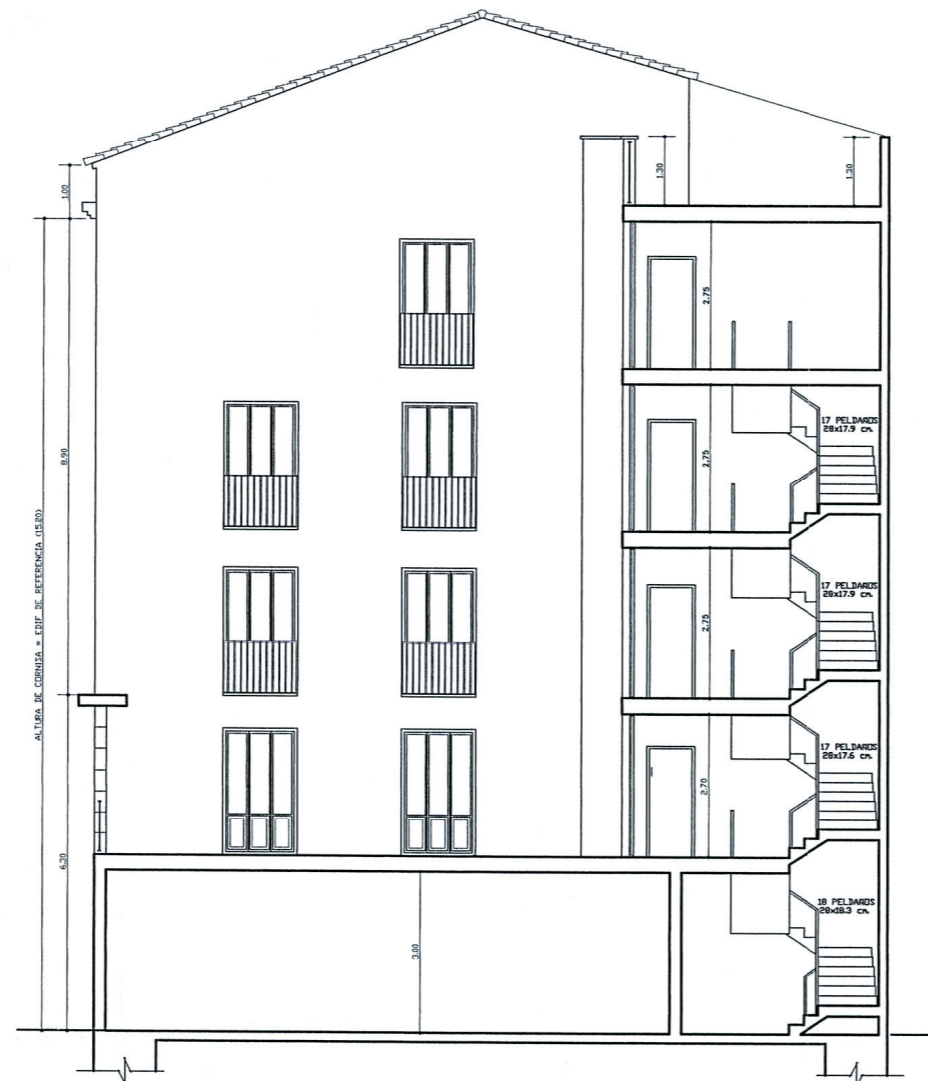
EDIF. E.D. SECCION 2-2
