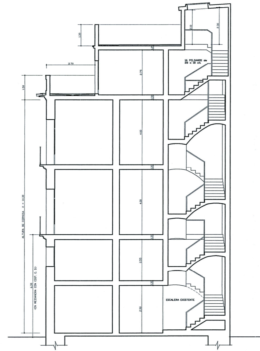
EDIF. PROT. NIVEL 2 SECCION 3-3
