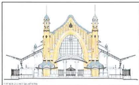
Alzado en la Calle Conde Salvatierra
