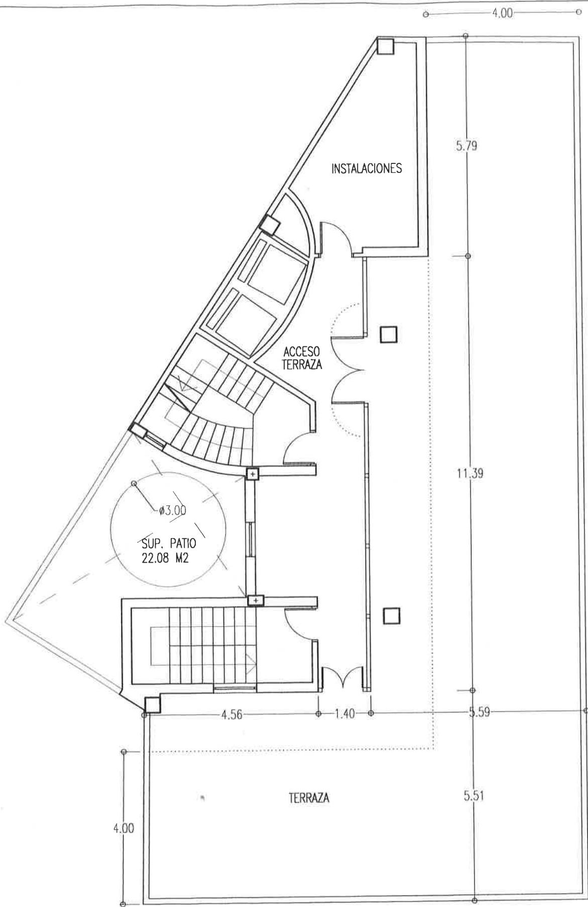
3.7. PLANTA CASETONES
