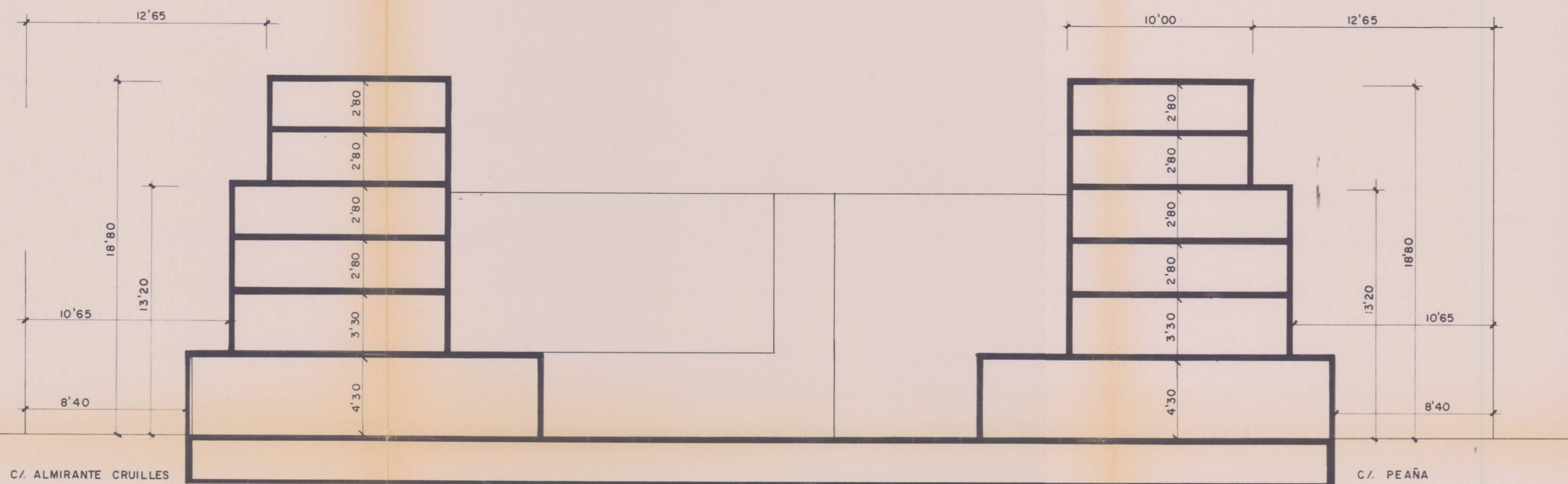
SECCION A-A'
