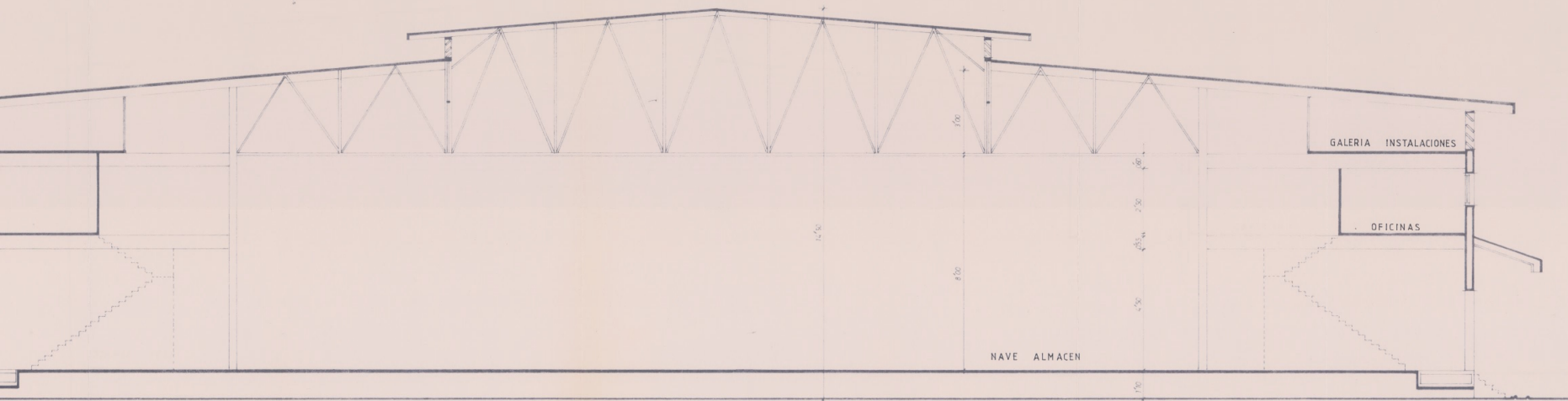
SECCION TRANSVERSAL B - B'
