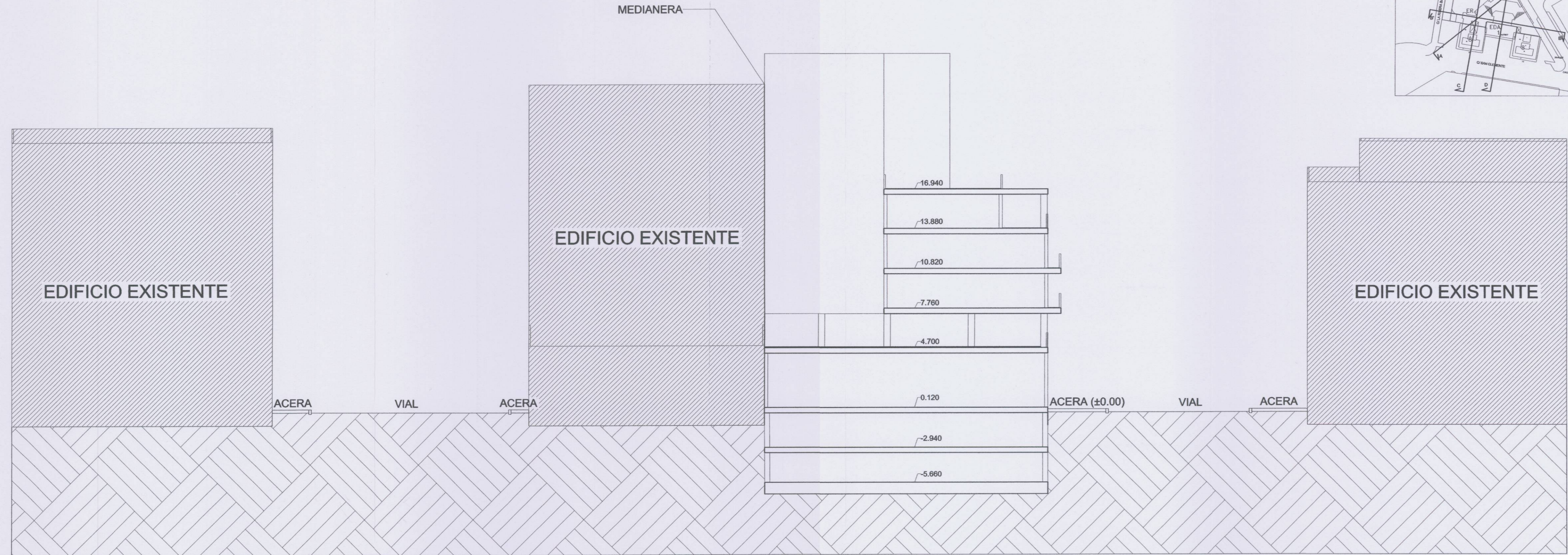
SECCIÓN D-D'
