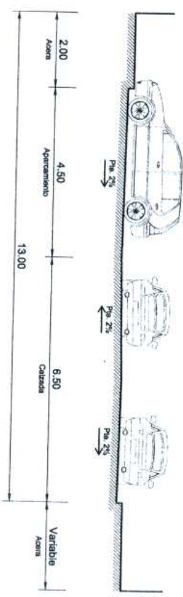
CALLE-D Nota: cotas en metros
