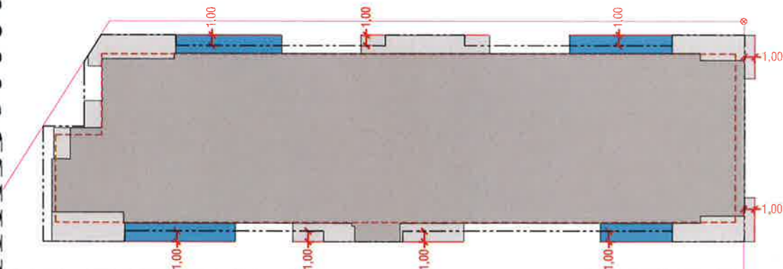
PLANTAS 2-4-6 sup. cerrada: 990,09 m 2 sup. abierta cubierta (50%) 62,30 m 2 sup. total: 1.052,39 m 2
