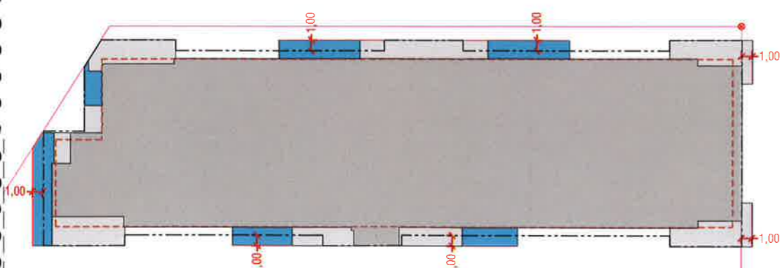
PLANTAS 3-5-7 sup. cerrada: 990,09 m 2 sup. abierta cubierta (50%) 62,30 m 2 sup. total: 1.052,39 m 2
