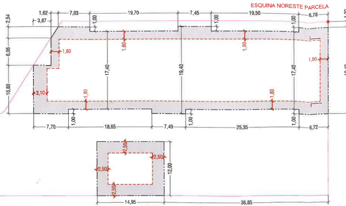
PLANTA BAJA
